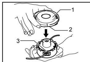
1. Couvercle 2. Saillie (n'est pas illustrée) 3. Encoche de l'œillet
